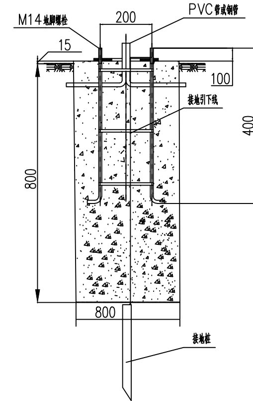
摄像机安装立杆地基、接地桩结构及安装图
