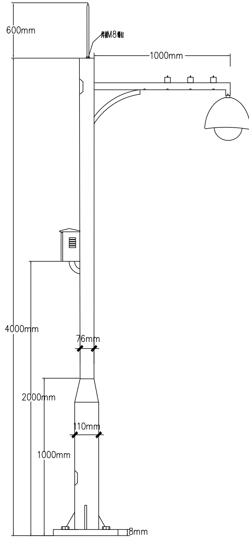
球型摄像机安装立杆剖面图
