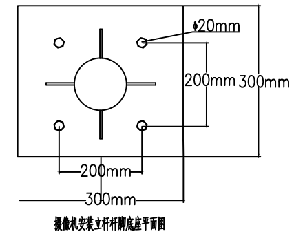
摄像机安装立杆底座平面图
